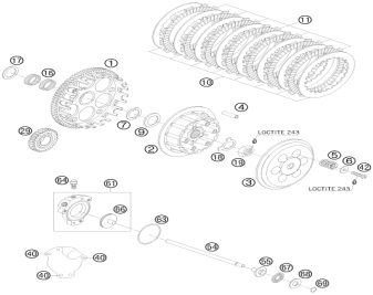
Clutch
