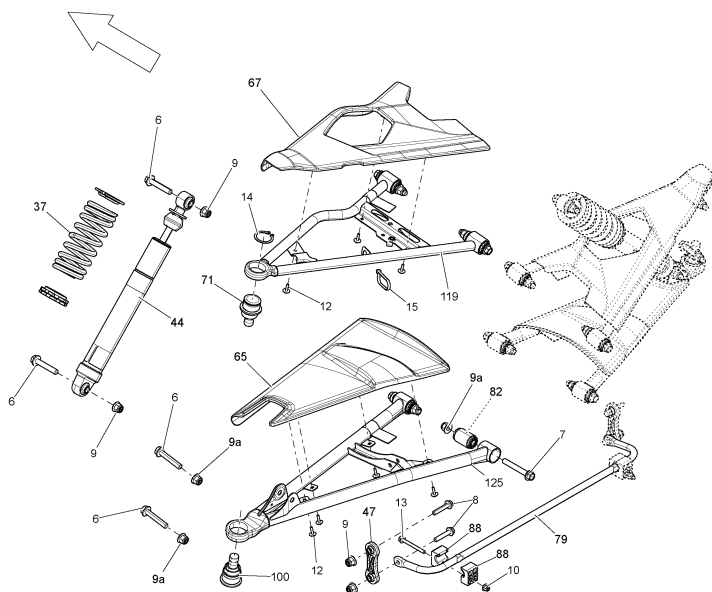
RS/RS-S/ST Model/Modèle, Common Parts/Pièces Communes
